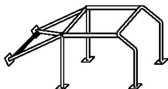
Dessin / No. 253-14 rajz
