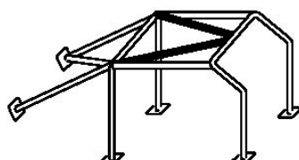
Dessin / No. 253-9B rajz
