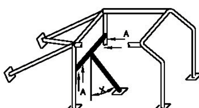
ⓧ Angle minimum 30° Minimális szög 30°
