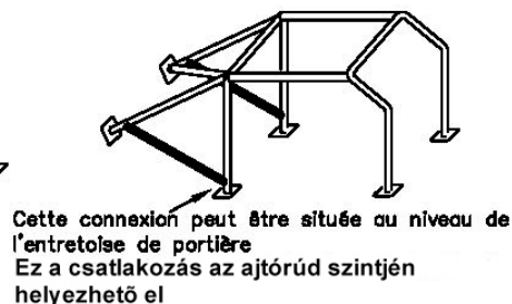
Dessin / No. 253-13 rajz
