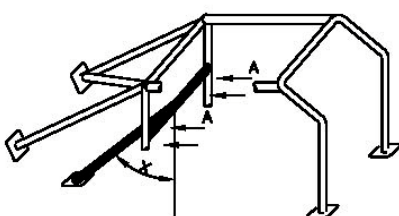
Ⓐ Trous de montage pour harnais Bekötőheveder szerelő furatai
