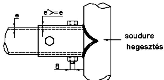
Dessin / No. 253-31 rajz
