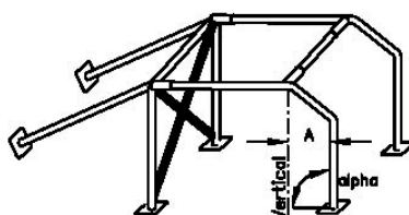
Dessin / No. 253-4 rajz
