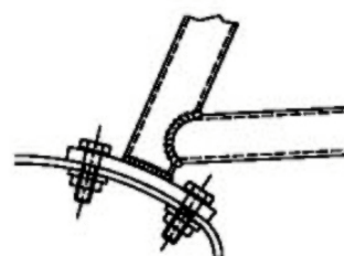
Dessin/ No. 253-25 rajz
