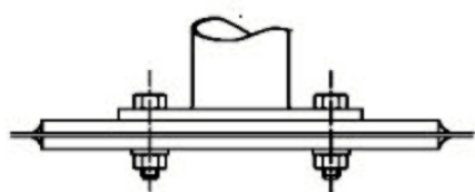
Dessin/ No. 253-20 rajz
