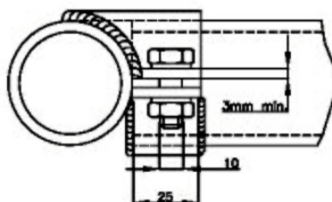
Dessin/ No. 253-27 rajz
