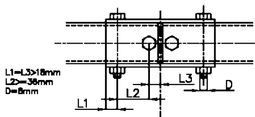
Dessin / No. 253-31 rajz
