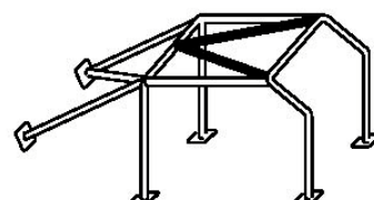
Dessin / No. 253-9C rajz
