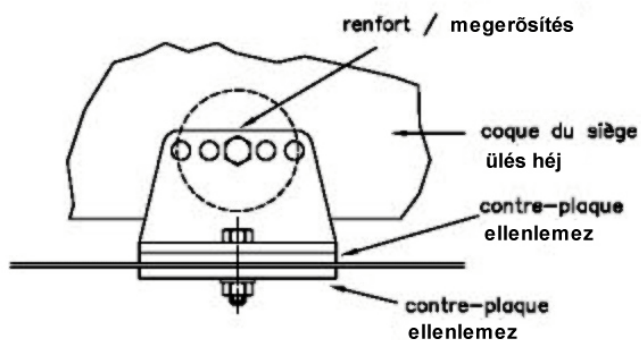
Dessin / No. 253-52 rajz
