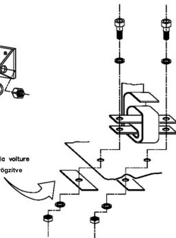
Dessin / No. 253-45 rajz
