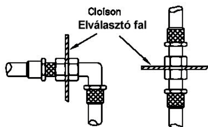
Dessin / No. 253-1 rajz
